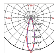
NLED317N 35W 24°
