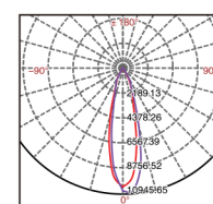
NLED317N 50W 24°
