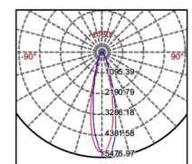
NLED5852A 2X9W 24°
