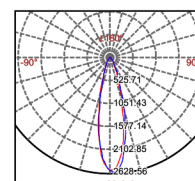
NMTLED5851A 9W 24°
